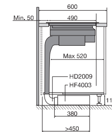
Zijaanzicht met liggend PlasmaMade filter en adapter
