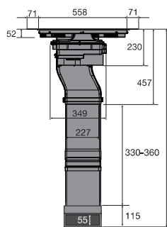
Vooraanzicht
