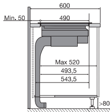
Zijaanzicht werkblad 600 mm
