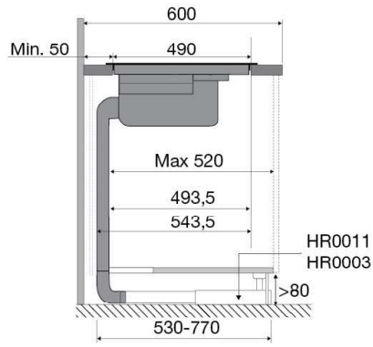
Zijaanzicht werkblad 600 mm Combinatie HR0003 en HR0011
