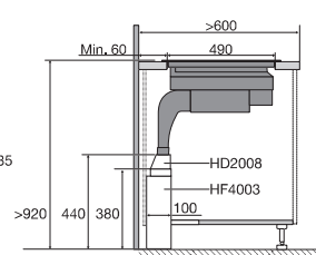
Zijaanzicht met PlasmaMade filter en adapter
