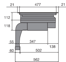
Zijaanzicht met PlasmaMade filter en adapter
