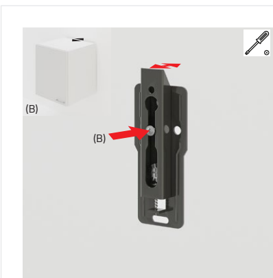
Diepteverstelling van hangkast met behulp van kruiskopschroevendraaier (B).
