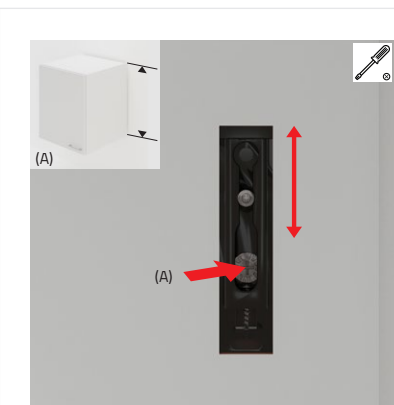
Hoogteverstelling van hangkast met behulp van kruiskopschroevendraaier (A).
